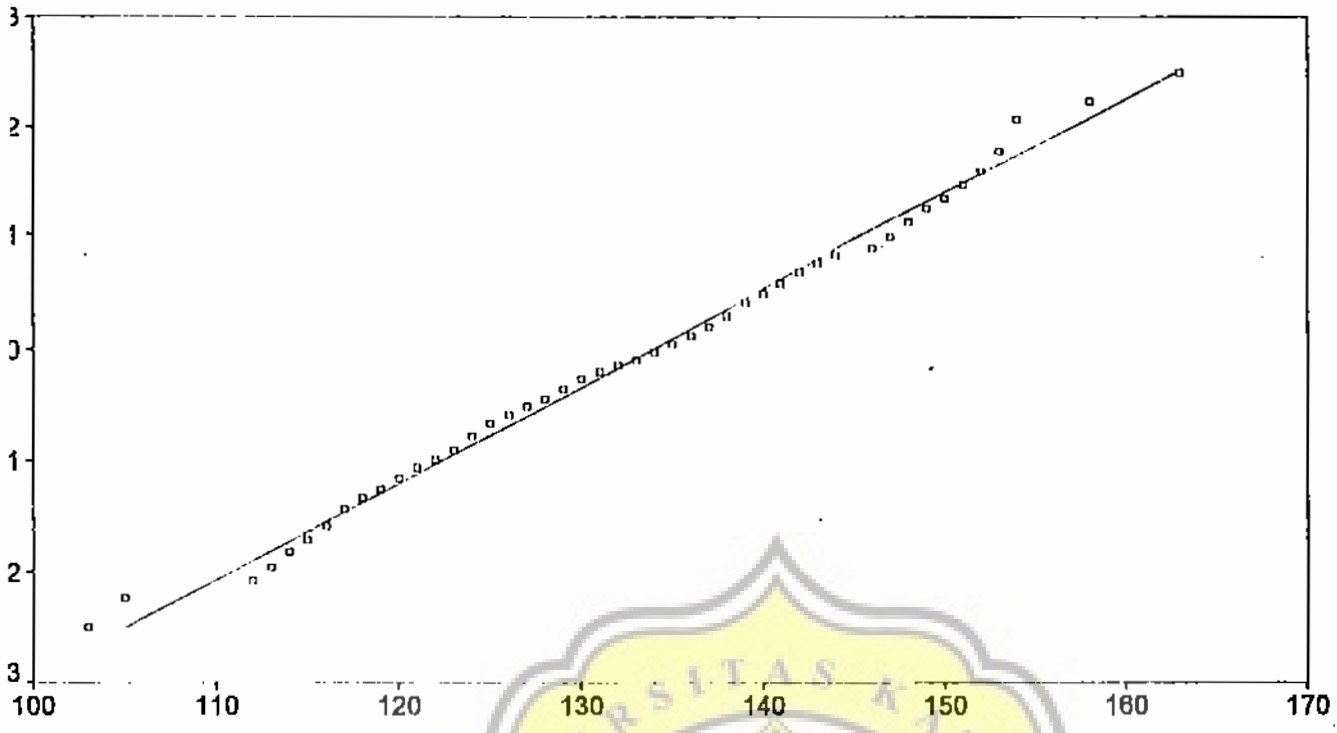
Normal Q-Q Plot of Persepsi terhadap Kepemimpinan Wanita pd Mhs Pria
