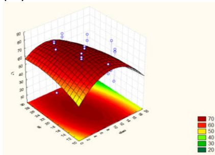
Gambar 27. Fitted response surface pengaruh penambahan oleoresin dan air terhadap warna ( L^* )
