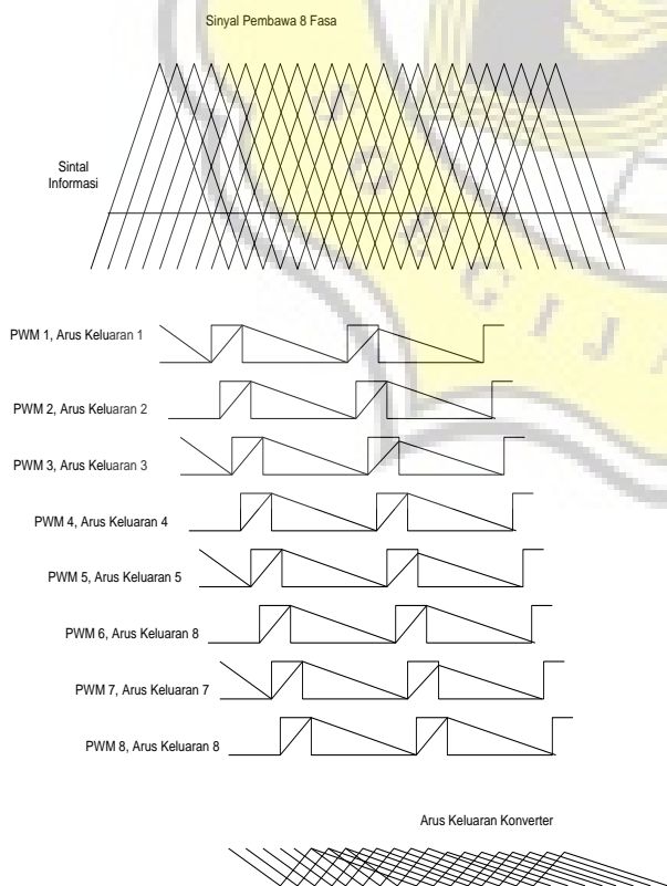
Gambar 4. Strategi kendali chopper delapan fasa
