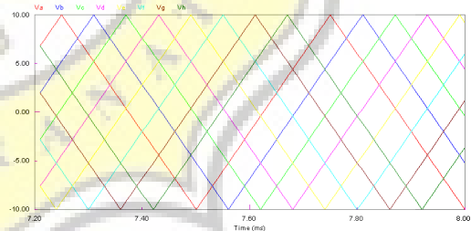
Gambar 9. Gelombang pembawa simulasi
