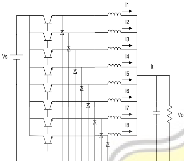
Gambar 3. Chopper delapan fasa
