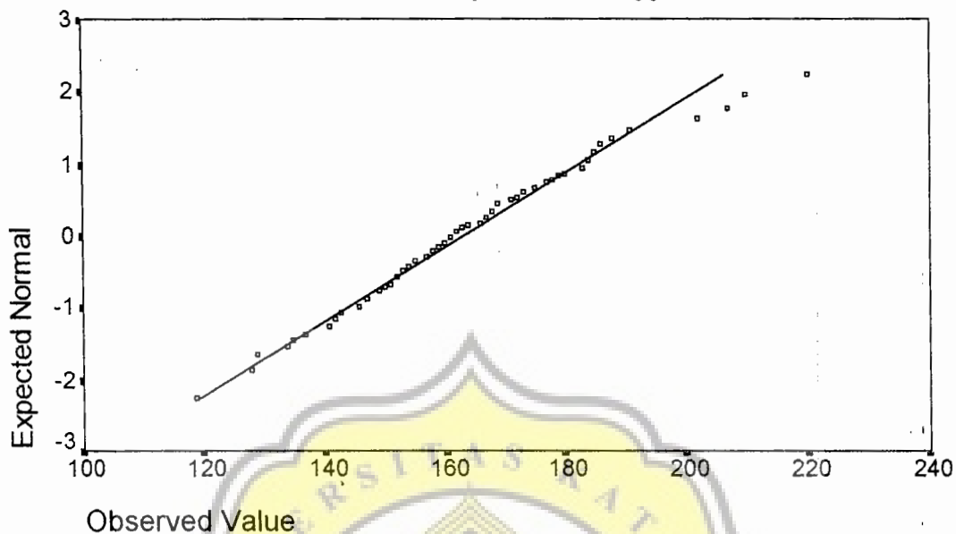
Normal Q-Q Plot of Motivasi Belajar Bahasa Inggris
