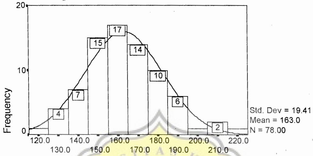
Motivasi Belajar Bahasa Inggris
