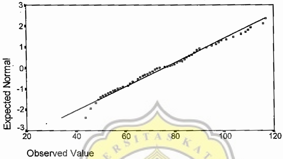
Normal Q-Q Plot of Kecemasan Berbicara diDepan Kelas
