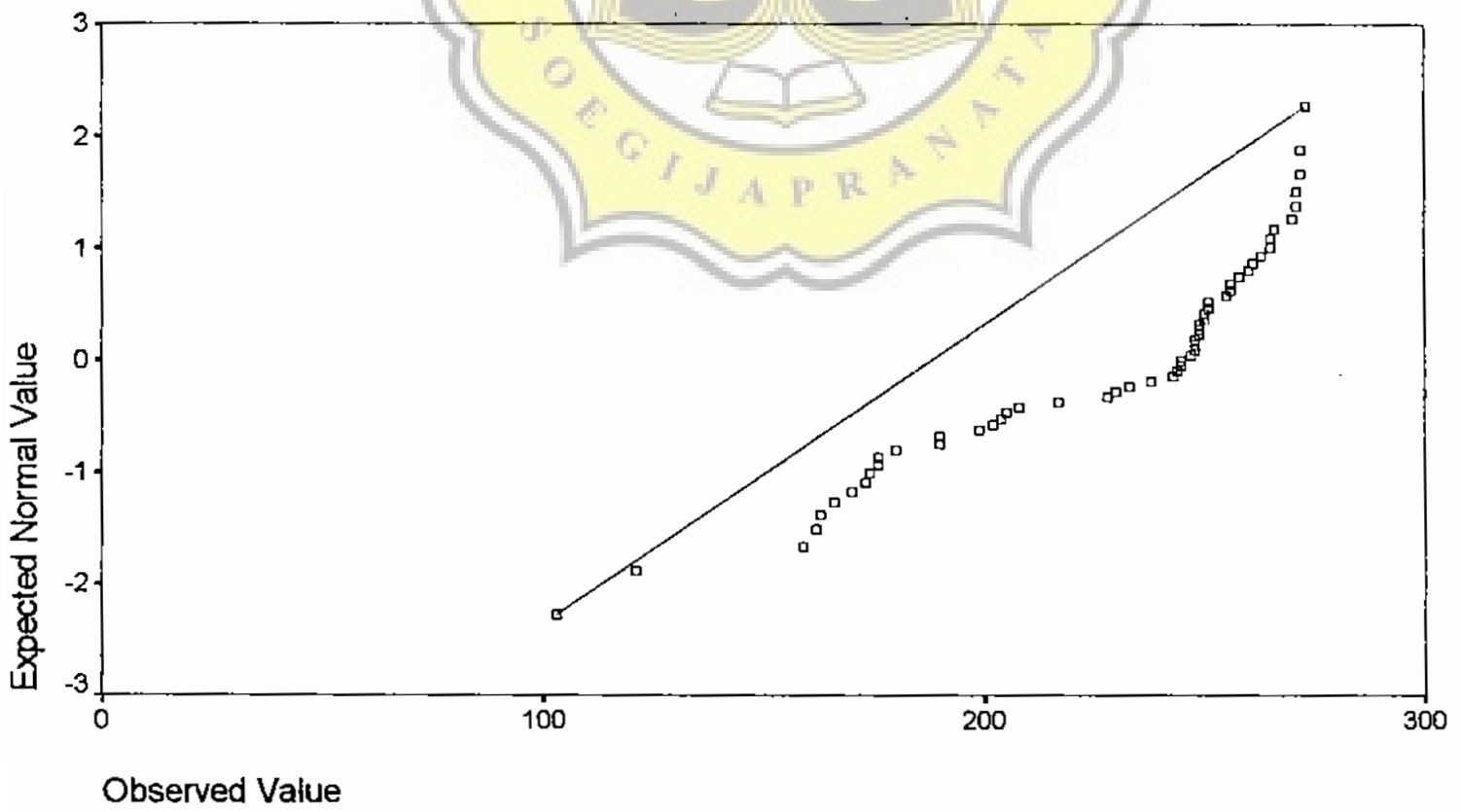
Normal Q-Q Plot of tingkat religiusitas
