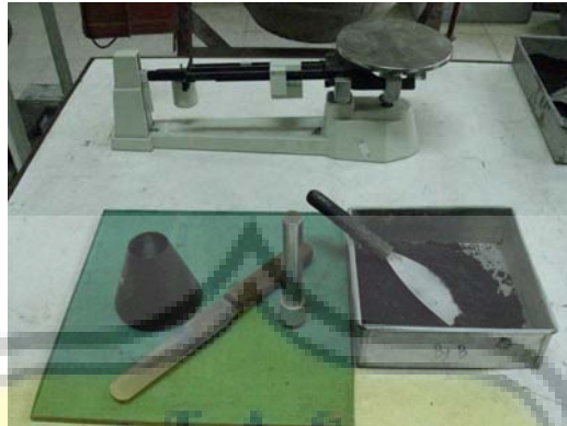
Alat-alat Uji Penyerapan Agregat Halus (Sumber: dokumentasi pribadi)
