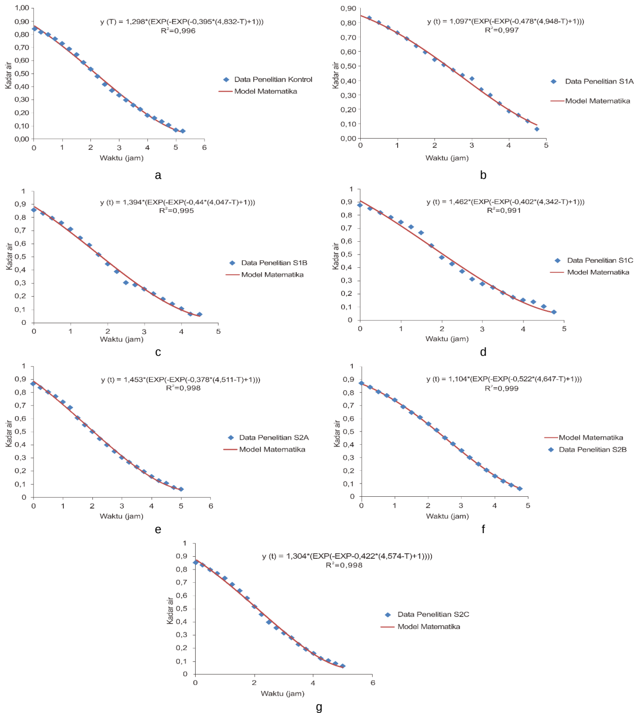
Gambar 3 Hubungan waktu pengeringan dan kadar air simplisia kunyit berdasarkan data penelitian dan model matematika (a) K, (b) S1A, (c) S1B, (d) S1C, (e) S2A, (f) S2B, dan (g) S2C.
