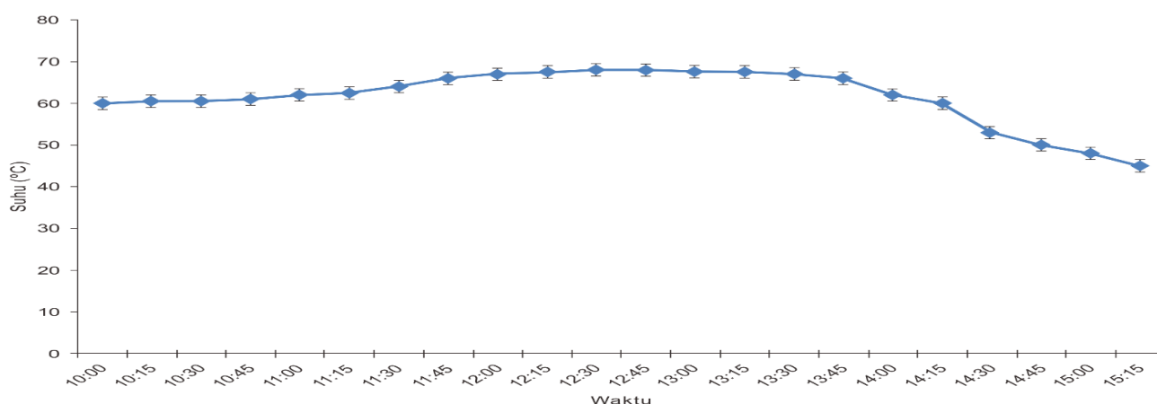
Gambar 2 Profil suhu solar tunnel dryer selama pengeringan.
