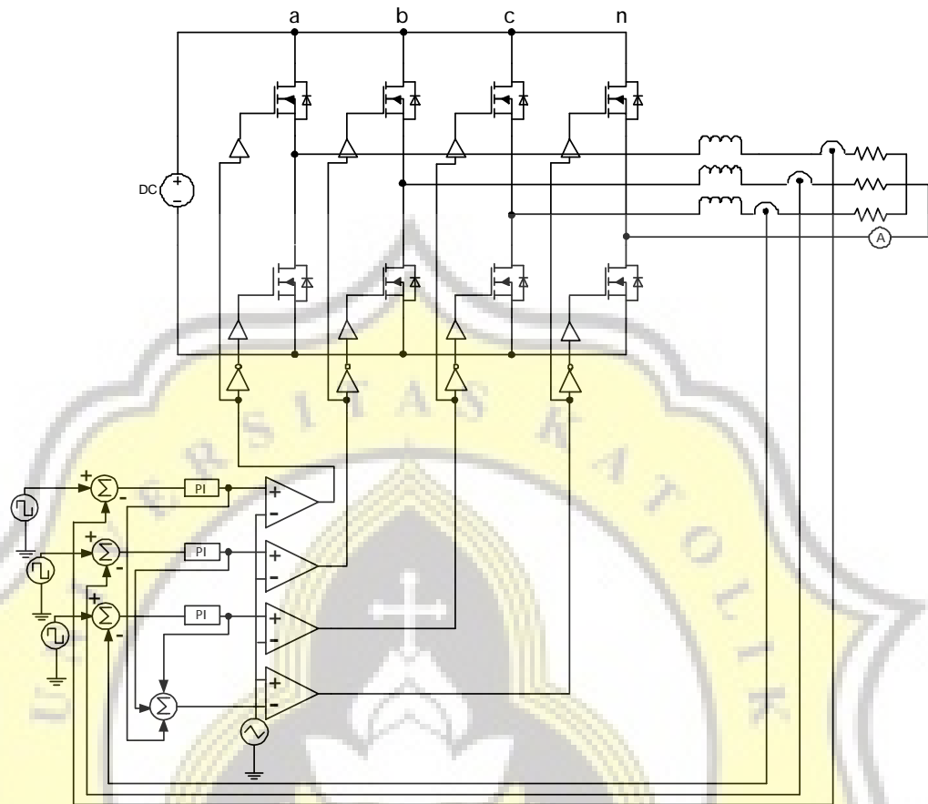
Gambar 2. Rangkaian Inverter Jenis Tegangan Tiga Fasa Empat Lengan Referensi Gelombang Kotak
