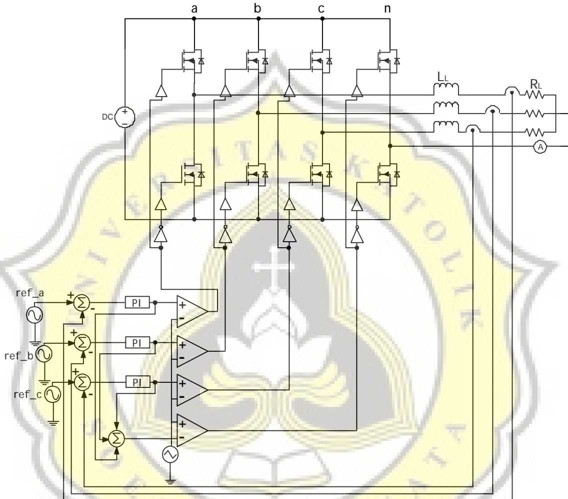
Gambar 4.3 Rangkaian Inverter Jenis Tegangan Tiga Fasa Empat Lengan Referensi Gelombang Sinusoidal
