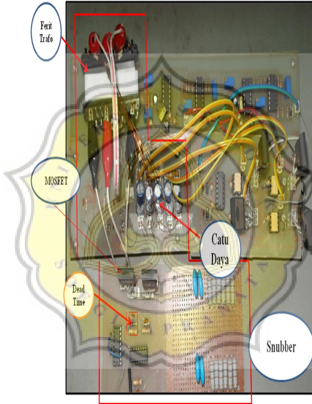
Gambar Rangkaian
