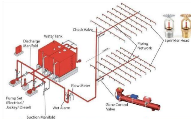
Gambar 6.8 Tataletak sprinkler wet riser
