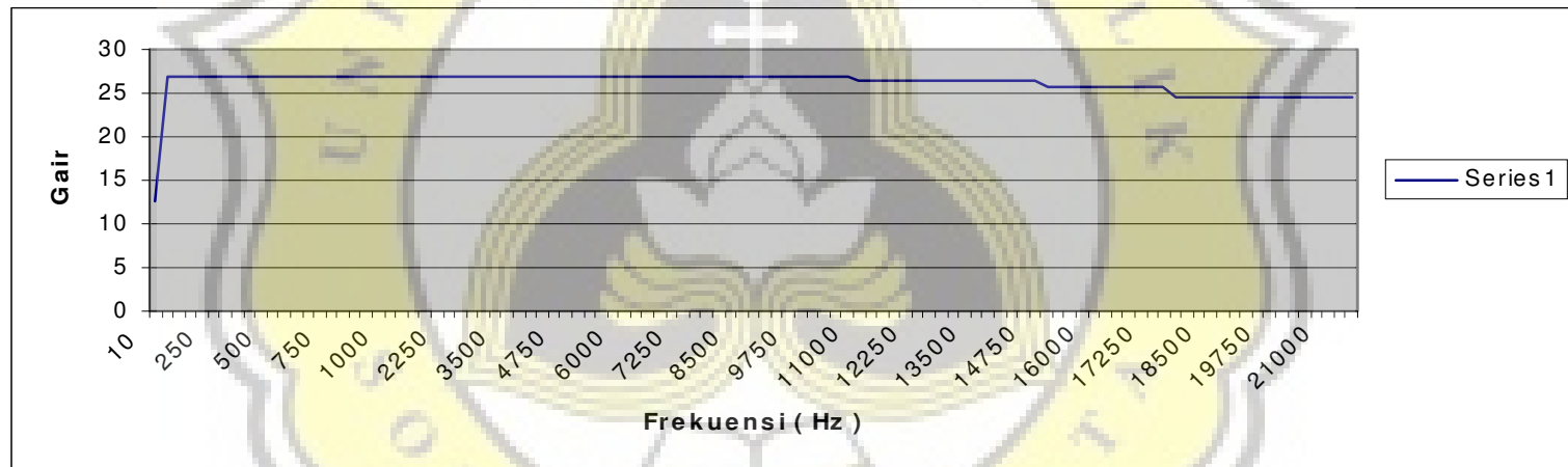
Gambar 3.9 Kurva Gain pada Power Amplifier
