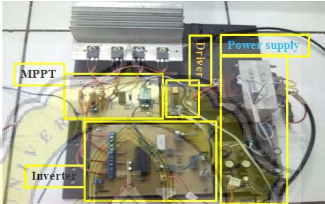
Gambar 1 Realisasi alat
