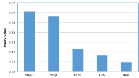
(b) tweetSanders, k=4
