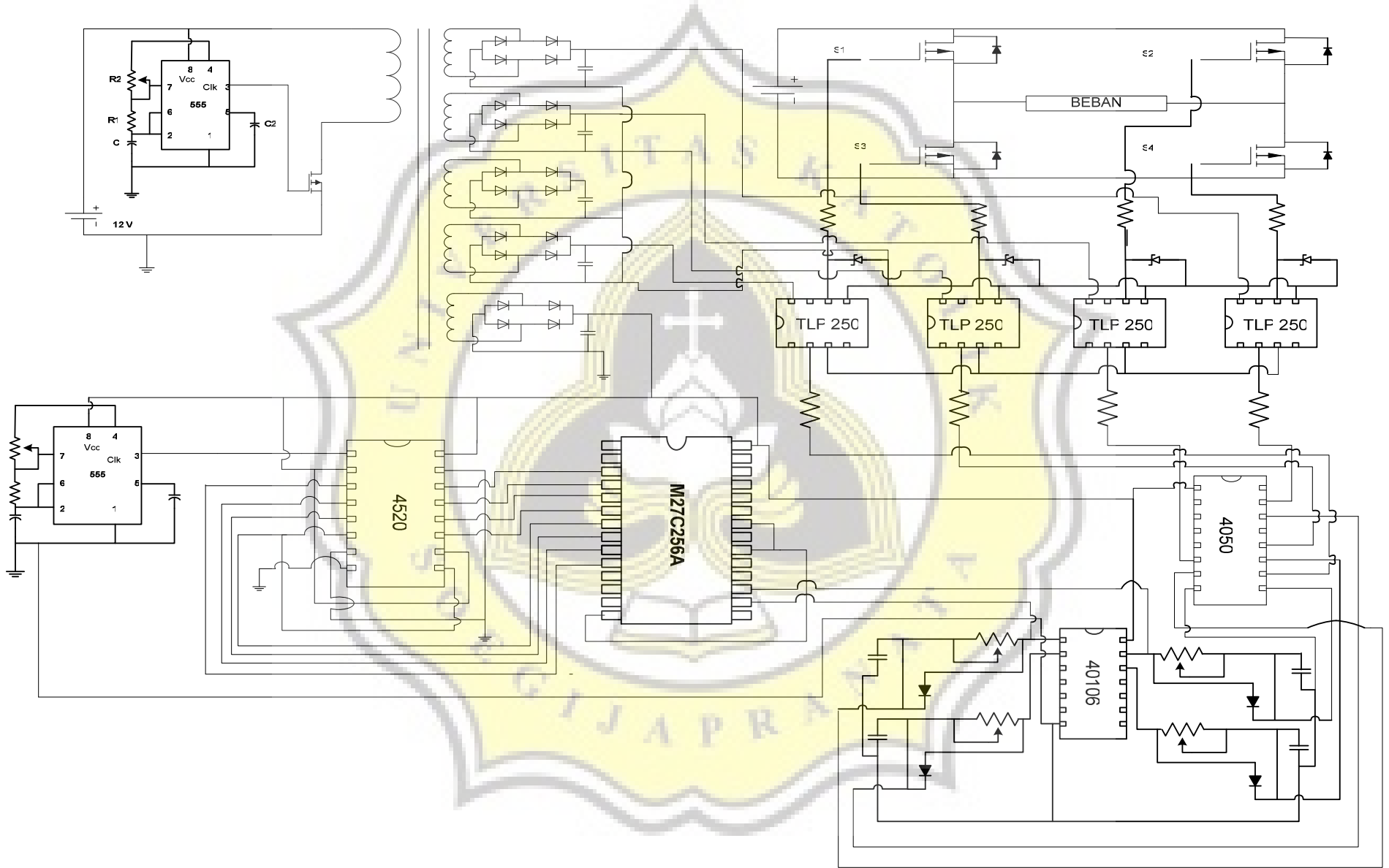
Gambar Lengkap DC – AC Konverter Kendali Digital
