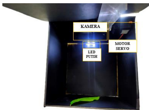
Gambar 3 Komponen dalam Kotak Hitam
