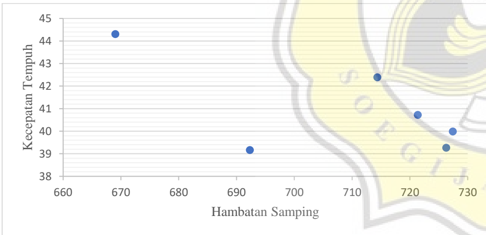
Grafik Hubungan Antara Volume Hambatan Sampung Dengan Kecepatan Tempuh Ruas Jalan Jendral Sudirman Pada Objek Sepeda Motor (Senin, 30 Mei 2022)
