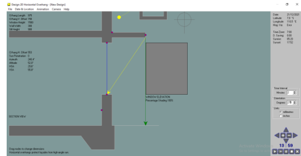
Shading panjang 1.00 m
