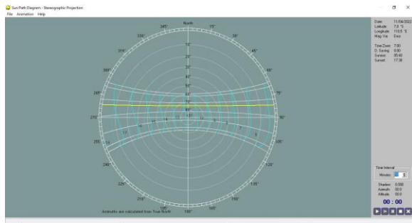
Gambar 3. Solar Chart kota Semarang
