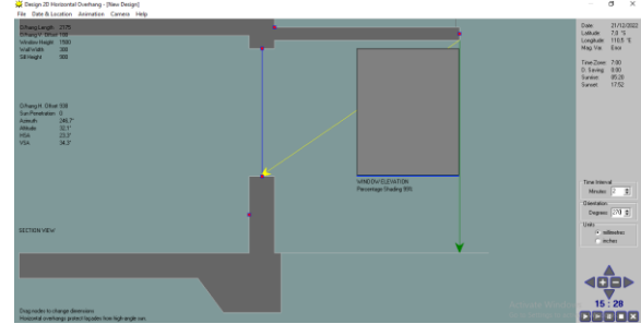
Shading panjang 2.00 m
