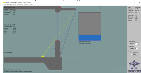
Sinar matahari masuk mulai jam 14.15 dengan sun shading panjang 1.00 m
