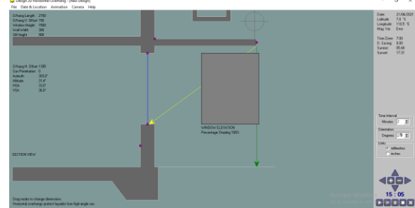
Sinar matahari masuk mulai jam 15.05 dengan sun shading panjang 2.00 m
