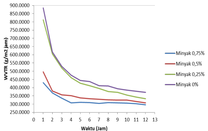
Figur 1. Karakter WVTR Edible Film Selama 12 Jam
