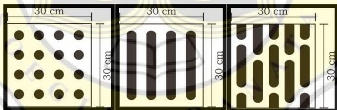
Tipe guiding block Sumber: Permen PUPR Nomor 14 Tahun 2017
