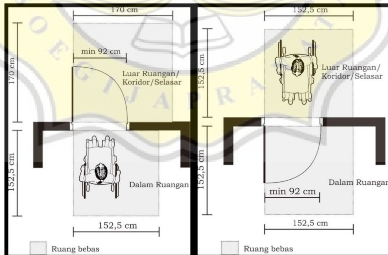
Lebar efektif pintu serta ruang bebas di dalam ruangan dan di luar ruangan/koridor/selasar Sumber: Permen PUPR Nomor 14 Tahun 2017
