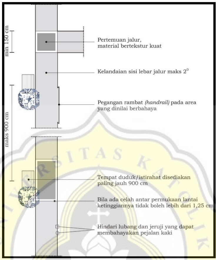
Prinsip perencanaan jalur pedestrian Sumber: Permen PUPR Nomor 14 Tahun 2017
