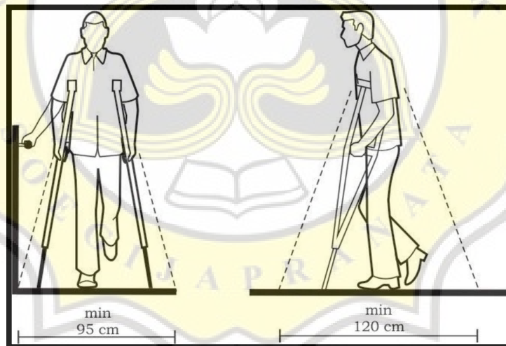
Jangkauan ke samping; ke depan dan ke belakang menggunakan kruk Sumber: Permen PUPR Nomor 14 Tahun 2017
