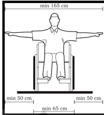
Jangkauan ke samping menggunakan 2 tangan pengguna kursi roda Sumber: Permen PUPR Nomor 14 Tahun 2017
