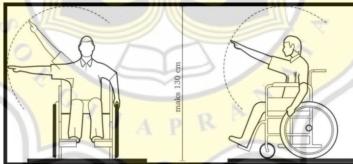
Jangkauan ke samping dan ke depan pengguna kursi roda
