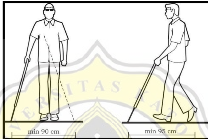
Jangkauan ke samping dan ke depan menggunakan tongkat Sumber: Permen PUPR Nomor 14 Tahun 2017
