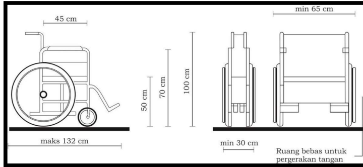
Tampak samping dan tampak depan kursi roda umum
