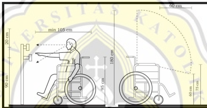
Jangkauan perletakan benda/peralatan dan jangkauan maksimal pengoperasian peralatan pengguna kursi roda Sumber: Permen PUPR Nomor 14 Tahun 2017
