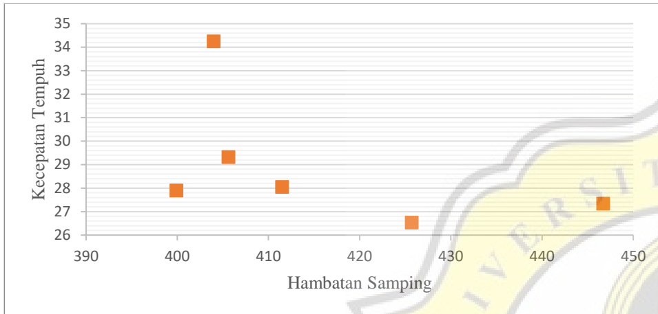
Grafik Hubungan Antara Volume Hambatan Samping Dengan Kecepatan Tempuh Ruas Jalan Ahmad Yani Pada Objek Kendaraan Ringan (Sabtu, 28 Mei 2022)
