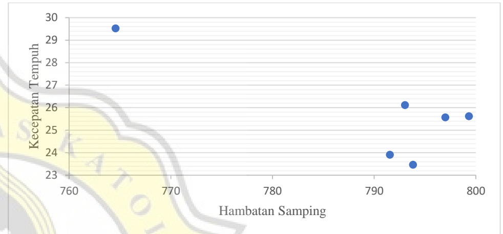
Grafik Hubungan Antara Volume Hambatan Samping Dengan Kecepatan Tempuh Ruas Jalan Jendral Sudirman Pada Objek Kendaraan Ringan (Minggu, 29 Mei 2022)
