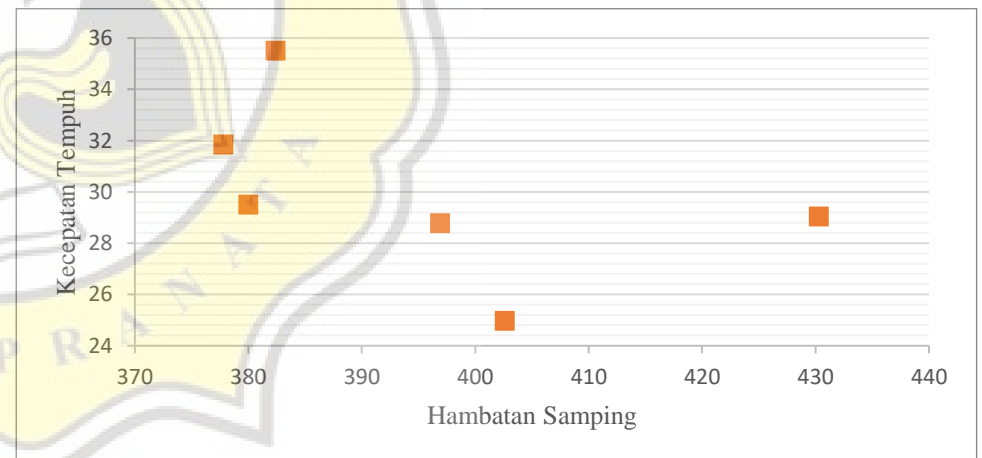
Grafik Hubungan Antara Volume Hambatan Samping Dengan Kecepatan Tempuh Ruas Jalan Ahmad Yani Pada Objek Kendaraan Ringan (Selasa, 31 Mei 2022)
