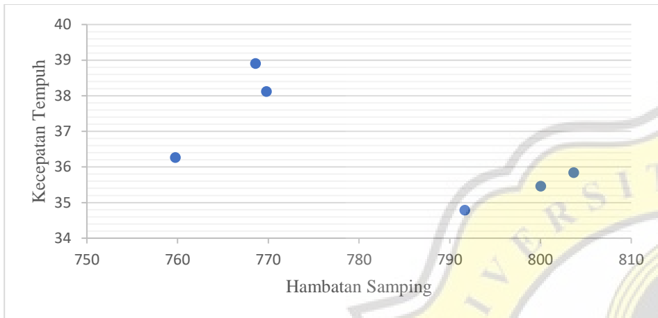
Grafik Hubungan Antara Volume Hambatan Sampung Dengan Kecepatan Tempuh Ruas Jalan Jendral Sudirman Pada Objek Sepeda Motor (Sabtu, 28 Mei 2022)
