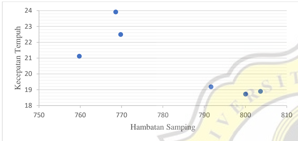
Grafik Hubungan Antara Volume Hambatan Samping Dengan Kecepatan Tempuh Ruas Jalan Jendral Sudirman Pada Objek Kendaraan Berat (Sabtu, 28 Mei 2022)
