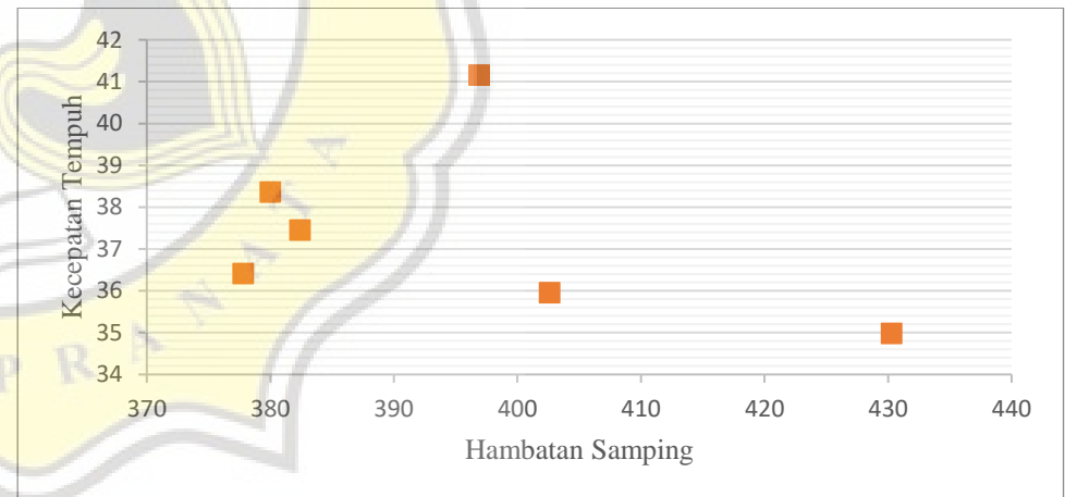
Grafik Hubungan Antara Volume Hambatan Samping Dengan Kecepatan Tempuh Ruas Jalan Ahmad Yani Pada Objek Sepeda Motor (Selasa, 31 Mei 2022)
