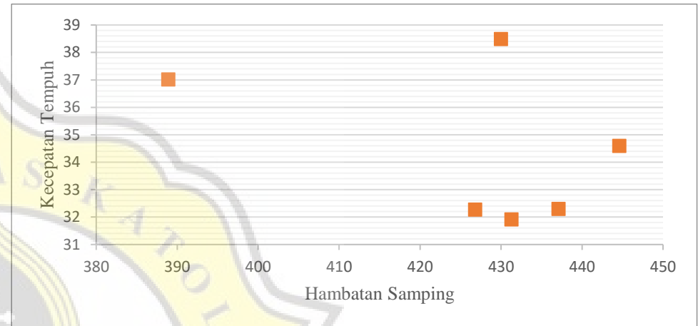
Grafik Hubungan Antara Volume Hambatan Samping Dengan Kecepatan Tempuh Ruas Jalan Ahmad Yani Pada Objek Sepeda Motor (Minggu, 29 Mei 2022)
