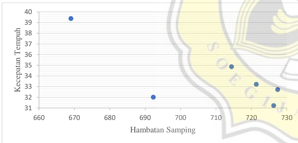
Grafik Hubungan Antara Volume Hambatan Samping Dengan Kecepatan Tempuh Ruas Jalan Jendral Sudirman Pada Objek Kendaraan Ringan (Senin, 30 Mei 2022)
