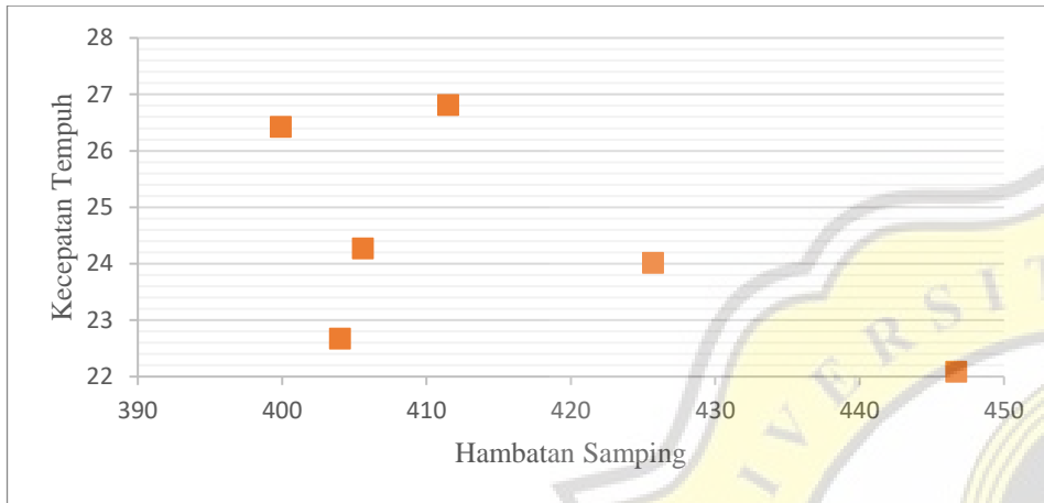
Grafik Hubungan Antara Volume Hambatan Samping Dengan Kecepatan Tempuh Ruas Jalan Ahmad Yani Pada Objek Kendaraan Berat (Sabtu, 28 Mei 2022)
