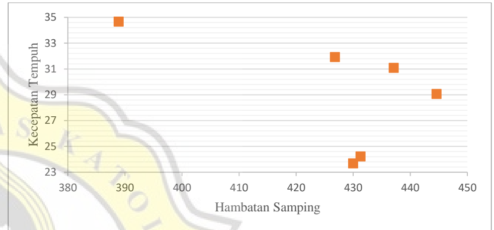
Grafik Hubungan Antara Volume Hambatan Samping Dengan Kecepatan Tempuh Ruas Jalan Ahmad Yani Pada Objek Kendaraan Ringan (Minggu, 29 Mei 2022)
