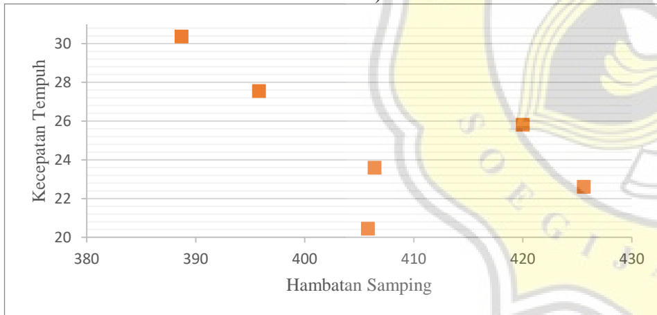
Grafik Hubungan Antara Volume Hambatan Samping Dengan Kecepatan Tempuh Ruas Jalan Ahmad Yani Pada Objek Kendaraan Berat (Senin, 30 Mei 2022)
