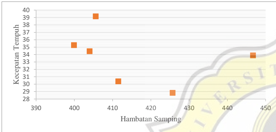
Grafik Hubungan Antara Volume Hambatan Samping Dengan Kecepatan Tempuh Ruas Jalan Ahmad Yani Pada Objek Sepeda Motor (Sabtu, 28 Mei 2022)
