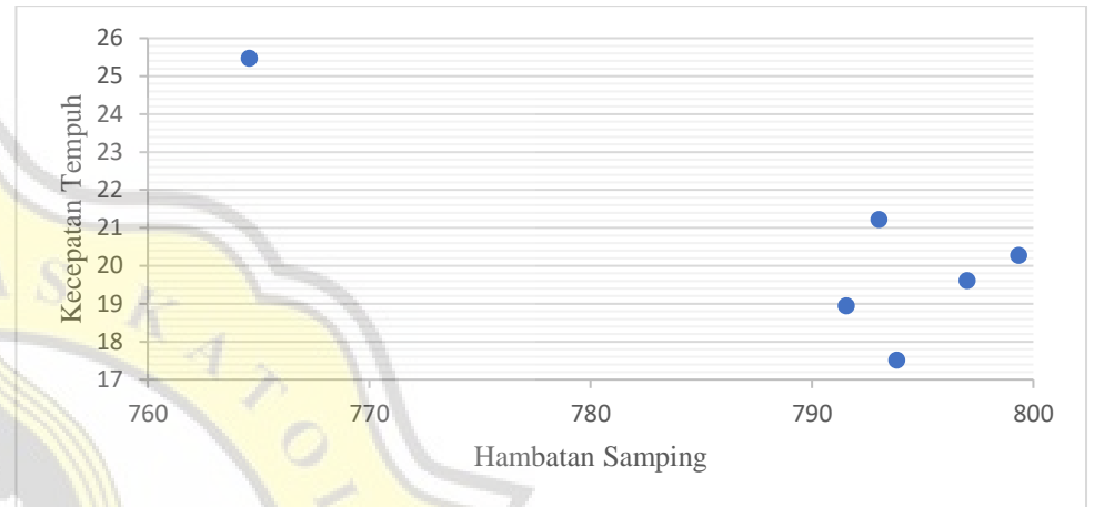
Grafik Hubungan Antara Volume Hambatan Samping Dengan Kecepatan Tempuh Ruas Jalan Jendral Sudirman Pada Objek Kendaraan Berat (Minggu, 29 Mei 2022)
