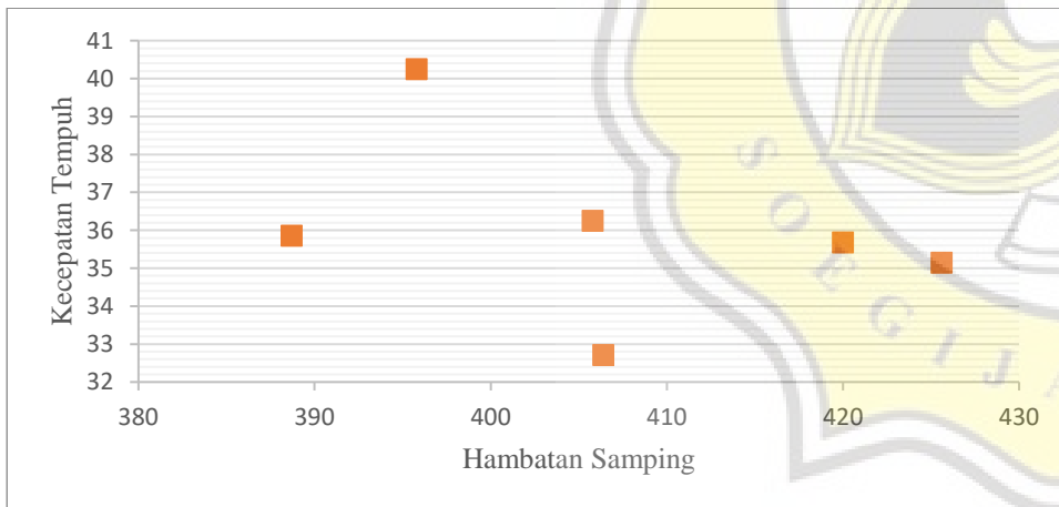
Grafik Hubungan Antara Volume Hambatan Samping Dengan Kecepatan Tempuh Ruas Jalan Ahmad Yani Pada Objek Sepeda Motor (Senin, 30 Mei 2022)
