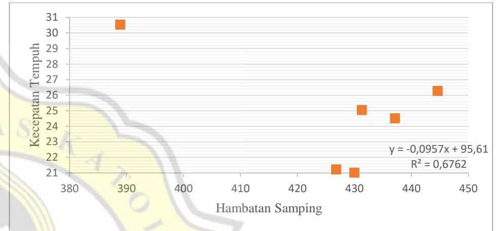
Grafik Hubungan Antara Volume Hambatan Samping Dengan Kecepatan Tempuh Ruas Jalan Ahmad Yani Pada Objek Kendaraan Berat (Minggu, 29 Mei 2022)
