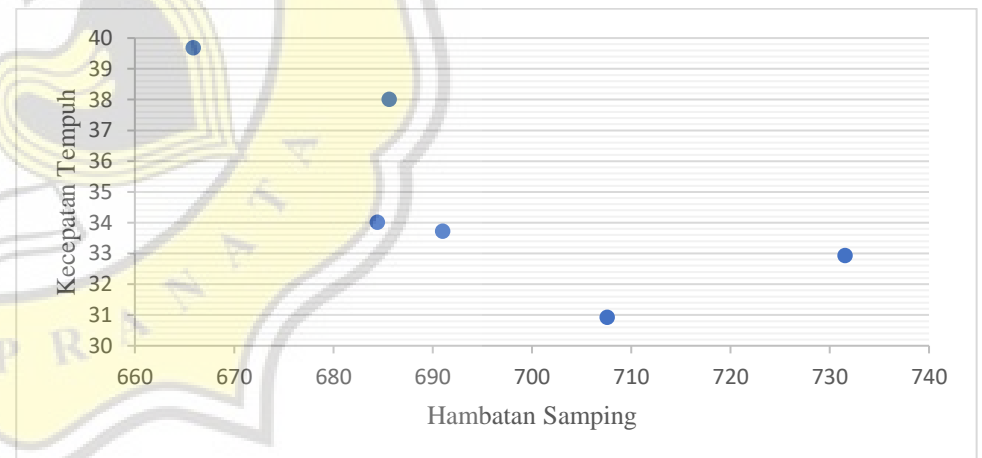
Grafik Hubungan Antara Volume Hambatan Samping Dengan Kecepatan Tempuh Ruas Jalan Jendral Sudirman Pada Objek Kendaraan Ringan (Selasa, 31 Mei 2022)
