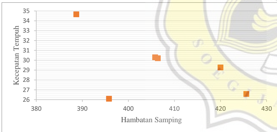
Grafik Hubungan Antara Volume Hambatan Samping Dengan Kecepatan Tempuh Ruas Jalan Ahmad Yani Pada Objek Kendaraan Ringan (Senin, 30 Mei 2022)
