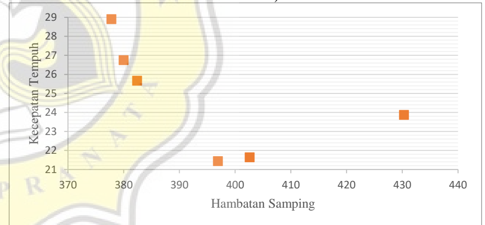
Grafik Hubungan Antara Volume Hambatan Samping Dengan Kecepatan Tempuh Ruas Jalan Ahmad Yani Pada Objek Kendaraan Berat (Selasa, 31 Mei 2022)
