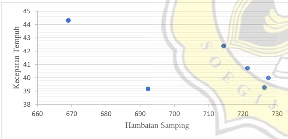
Grafik Hubungan Antara Volume Hambatan Sampung Dengan Kecepatan Tempuh Ruas Jalan Jendral Sudirman Pada Objek Sepeda Motor (Senin, 30 Mei 2022)
