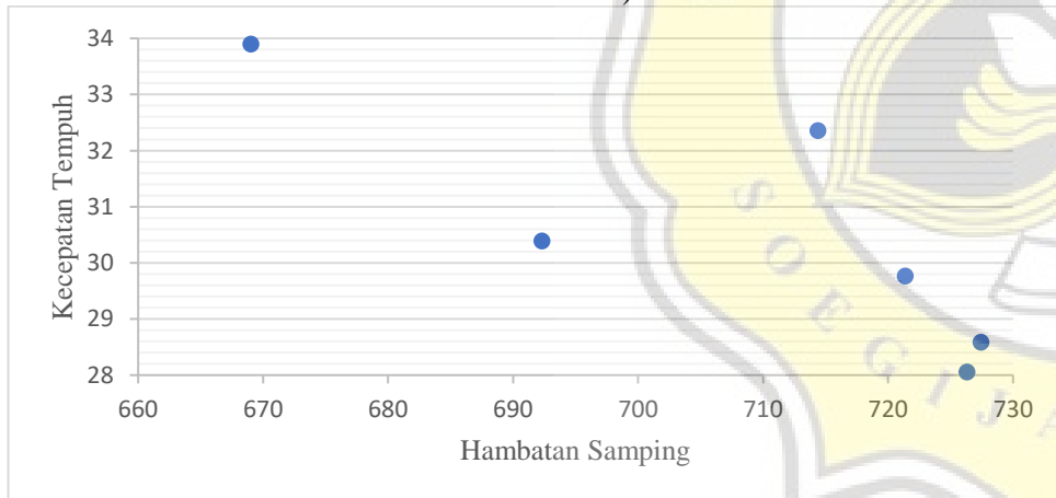
Grafik Hubungan Antara Volume Hambatan Samping Dengan Kecepatan Tempuh Ruas Jalan Jendral Sudirman Pada Objek Kendaraan Berat (Senin, 30 Mei 2022)
