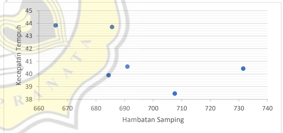
Grafik Hubungan Antara Volume Hambatan Sampung Dengan Kecepatan Tempuh Ruas Jalan Jendral Sudirman Pada Objek Sepeda Motor (Selasa, 31 Mei 2022)
