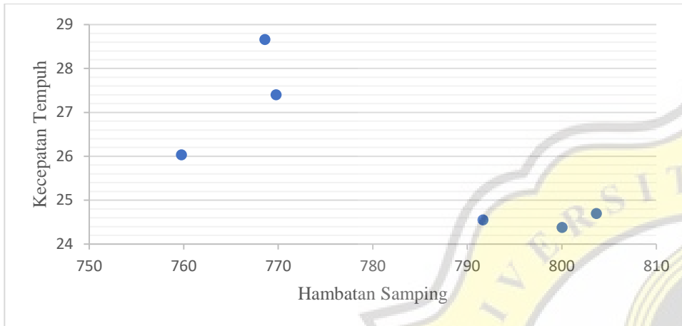
Grafik Hubungan Antara Volume Hambatan Samping Dengan Kecepatan Tempuh Ruas Jalan Jendral Sudirman Pada Objek Kendaraan Ringan (Sabtu, 28 Mei 2022)
