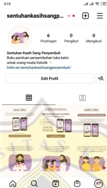
Gambar 42. Profil Instagram
