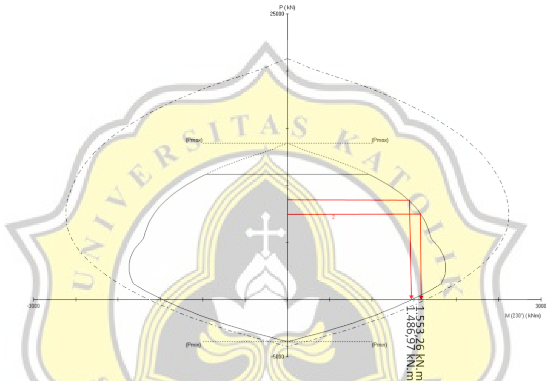
Gambar 4.19 Diagram Interaksi Kolom K1 Lantai 2 dan Lantai 3
