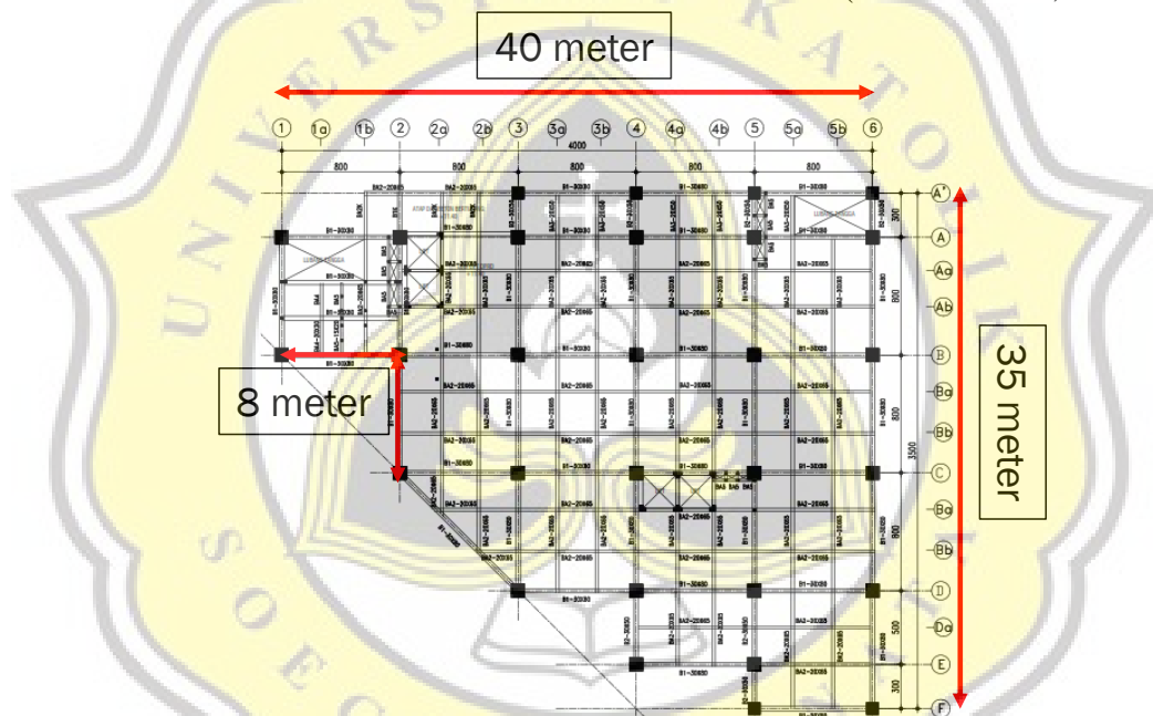
Gambar 4.3 Pemeriksaan Ketidakberaturan Sudut Dalam
