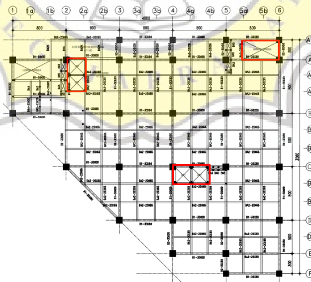
Gambar 4.5 Pemeriksaan Ketidakberaturan Diskontinuitas Diafragma
