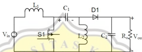
Gambar 1. Rangkaian Ekuivalen Konvensional SEPIC Konverter
