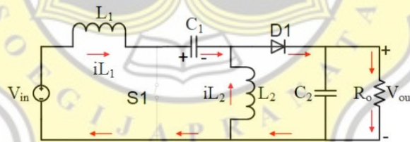
Gambar 3. Mode Operasi SEPIC Konverter Konvensional saat Saklar OFF
