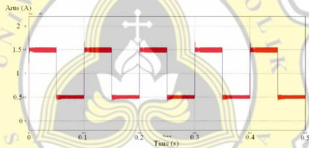
Gambar 8. Aktual dan Referensi pada Simulasi PSIM
