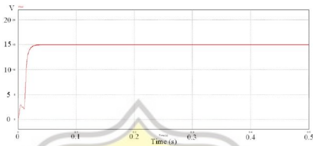
Gambar 10. Tegangan Keluaran SEPIC Konverter dengan Referensi 1.5 A pada Simulasi PSIM
