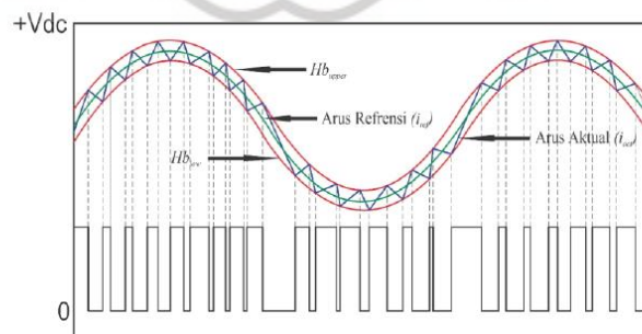
Gambar 4. Pita Histeresis pada Sistem Kendali Arus Histeresis
