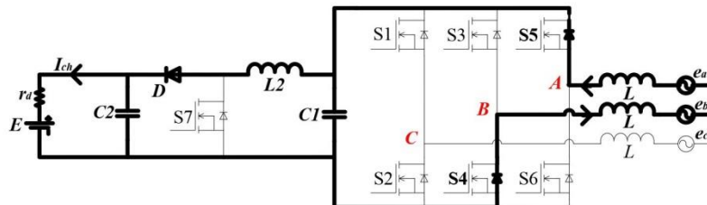
Gambar 6. Rangkaian ekivalen pengereman regeneratif mesin BLDC saat energi pada belitan mengalir melalui dioda (Riyadi dkk., 2019)
