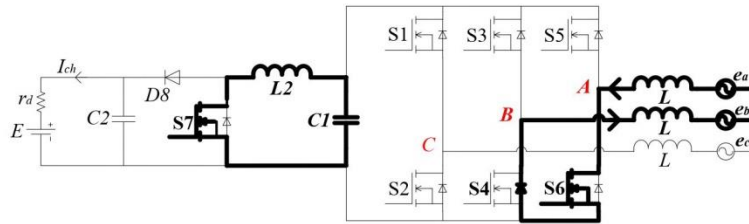
Gambar 4. Rangkaian ekivalen pengereman regeneratif mesin BLDC pada saat belitan menyimpan energi (Riyadi dkk., 2019)
