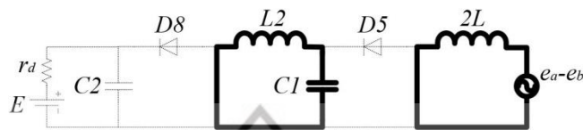
Gambar 5. Rangkaian ekivalen cascaded boost converter ketika saklar dalam kondisi-on (Riyadi dkk., 2019)
