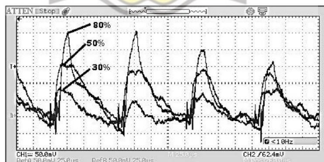
Gambar 14. Hasil percobaan perbandingan arus yang masuk ke batere ( I_{ch} ) saat duty cycle (a) 0,3 (b) 0,5 (c) 0,8
