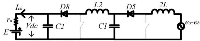
Gambar 7. Rangkaian ekivalen cascaded boost converter saat saklar dalam kondisi- off (Riyadi dkk., 2019)
