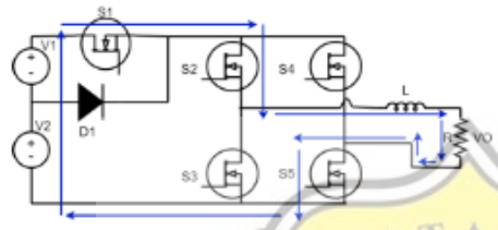
Gambar 4. Mode operasi satu, saat sakelar S1 , S2 , dan S5 konduksi
