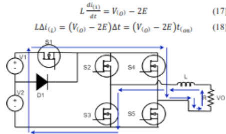
Gambar 8. Mode operasi lima, saat sakelar S1, S3, dan S4 konduksi
