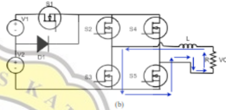
Gambar 6. Mode operasi tiga, (a) siklus positif, saat sakelar S2 dan S4 konduksi, (b) siklus negatif, saat sakelar S3 dan S5 konduksi
