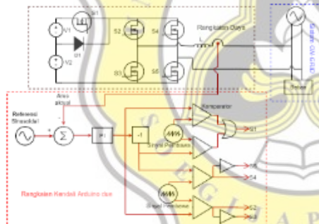
Gambar 9. Blok diagram sistem kendali inverter lima tingkat
