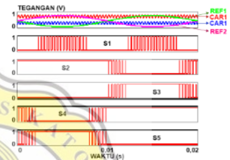
Gambar 10. Bentuk sinyal pensakelaran pada tiap sakelar daya
