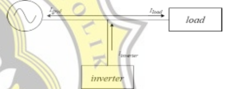
Gambar 2. Pengiriman arus inverter pada sistem on-grid
