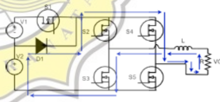
Gambar 7. Mode operasi empat, saat sakelar S3 dan S4 konduksi
