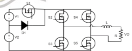
Gambar 3. Topologi rangkaian inverter lima tingkat
