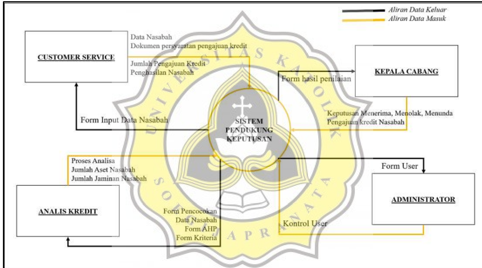
Gambar 4.1 Diagram Konteks
