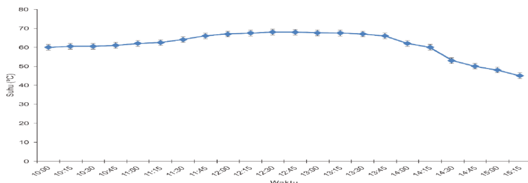
Gambar 2 Profil suhu solar tunnel dryer selama pengeringan.
