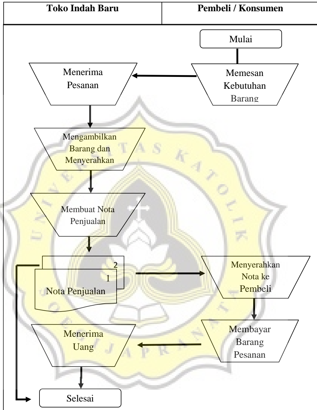
Gambar 3 Flowchart Sistem Penjualan Toko Indah Baru
