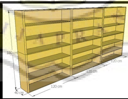
Dimensi Rak Buku Sumber : Analisa Pribadi
