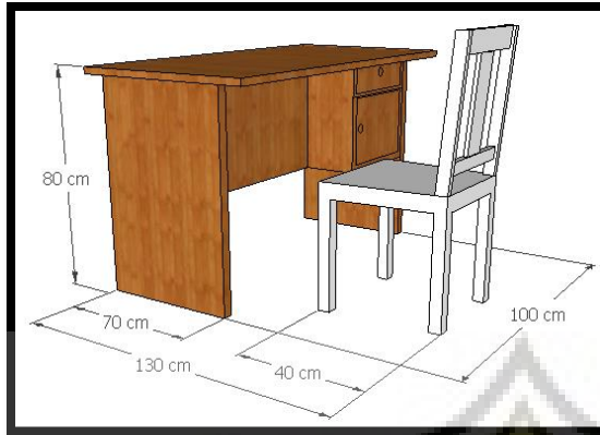
Dimensi Meja Belajar Sumber : Analisa Pribadi
