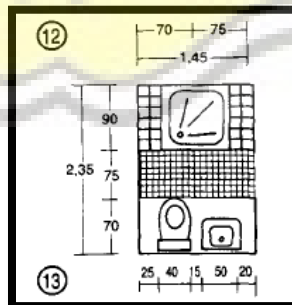
Denah Kamar Mandi Anak Sumber : Analisa Pribadi
