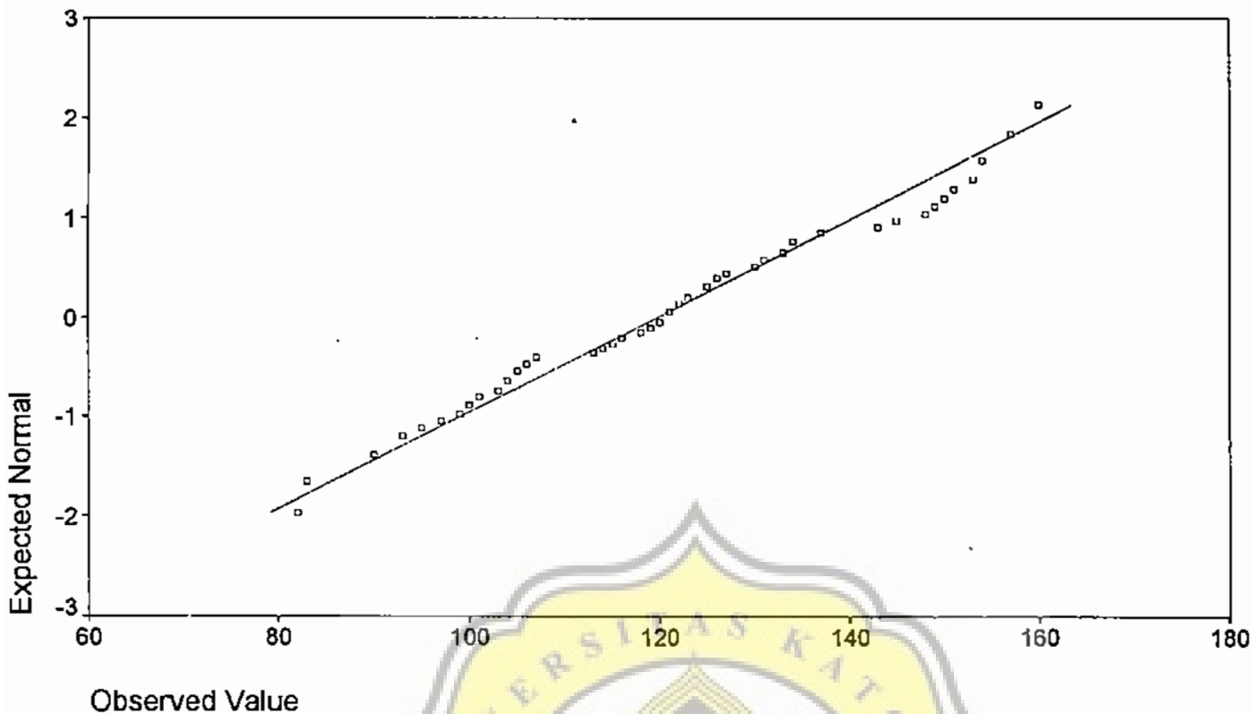
Normal Q-Q Plot of Sikap Remaja terhadap Hubungan Seks Pranikah (Laki-la
