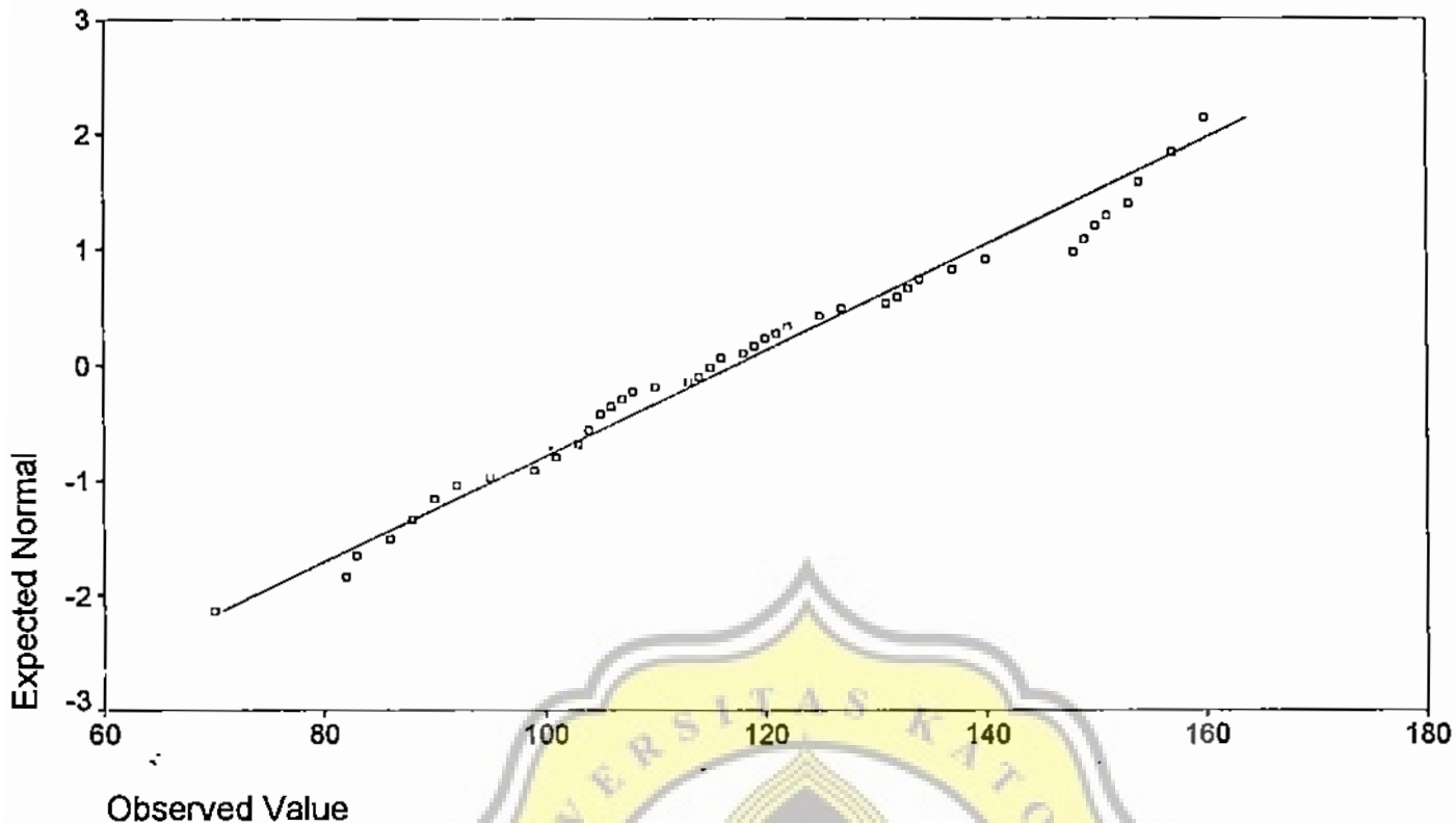
Normal Q-Q Plot of Sikap Remaja terhadap Hubungan Seks Pranikah (Kota)
