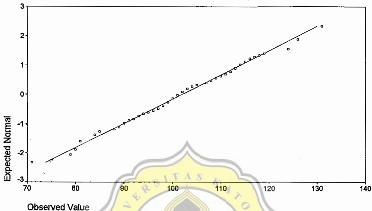
Normal Q-Q Plot of Kecenderungan Agresi Wanita Tengah Baya
