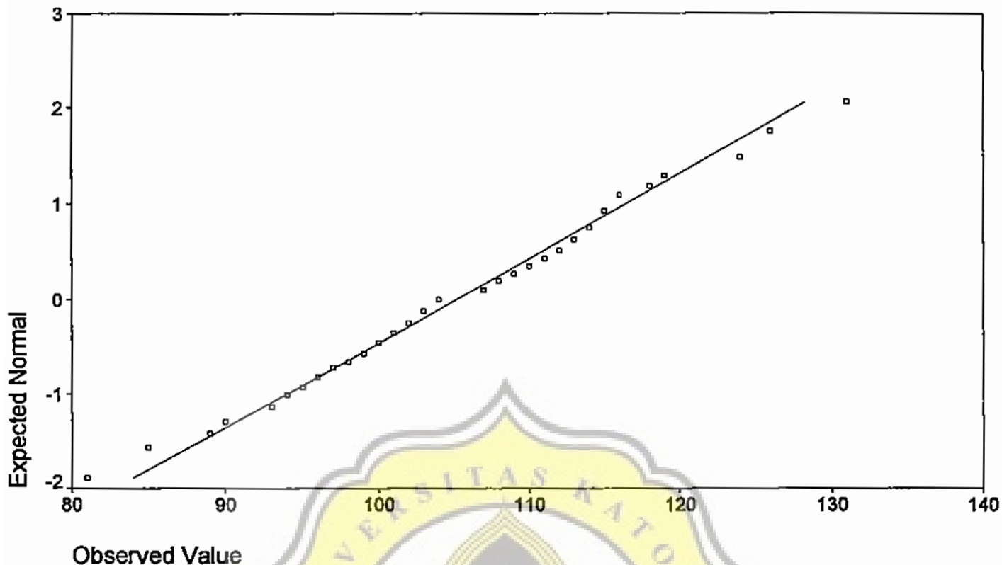
Normal Q-Q Plot of Kecenderungan Agresi Wanita Tengah Baya (Rumah Susun)
