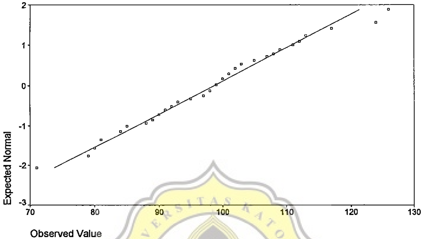
Normal Q-Q Plot of Kecenderungan Agresi Wanita Tengah Baya (Rumah Tungga
