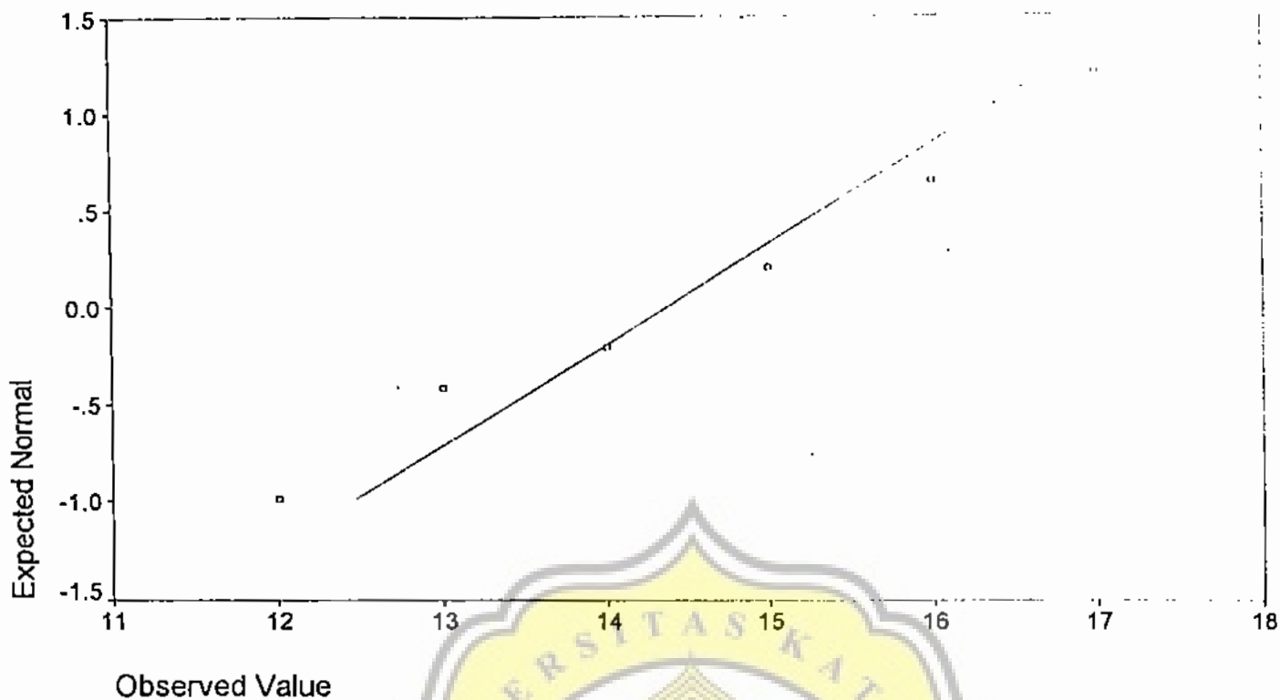
Normal Q-Q Plot of Tingkat Pendidikan
