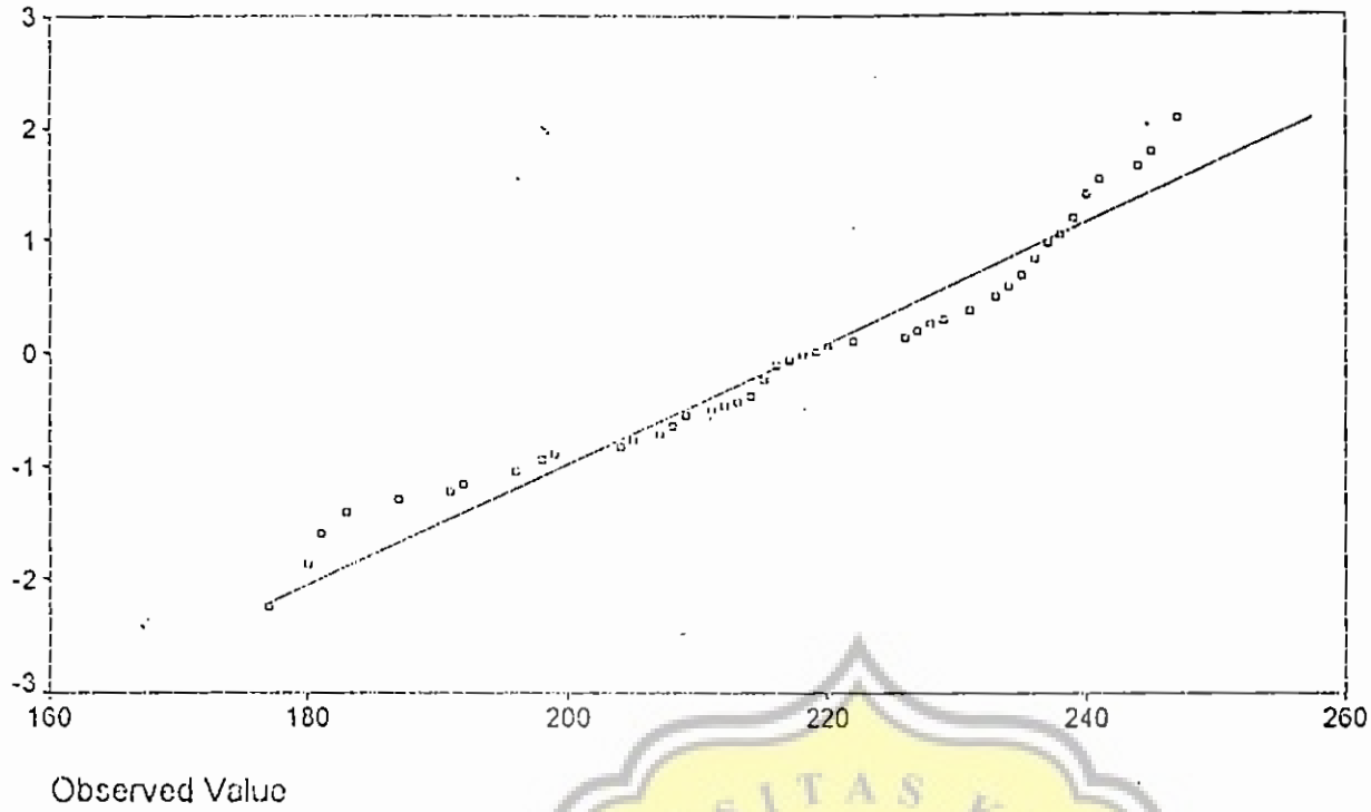
Normal Q-Q Plot of Tingkat Religiusitas
