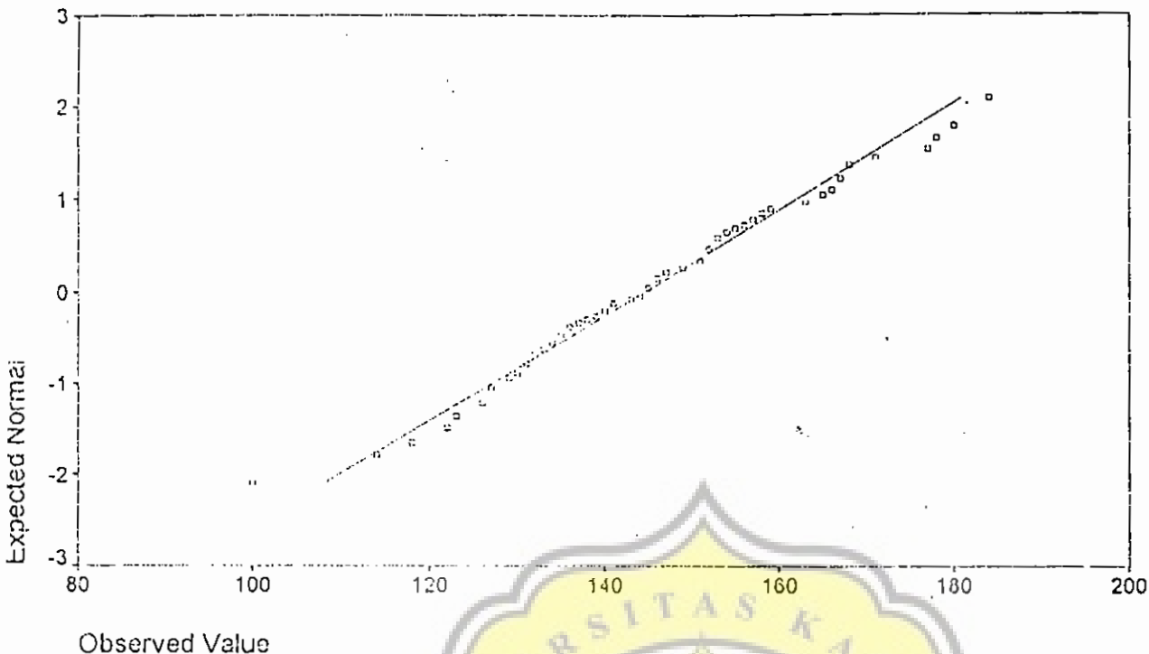
Normal Q-Q Plot of Kecemasan terhadap Perilaku Seksual Remaja
