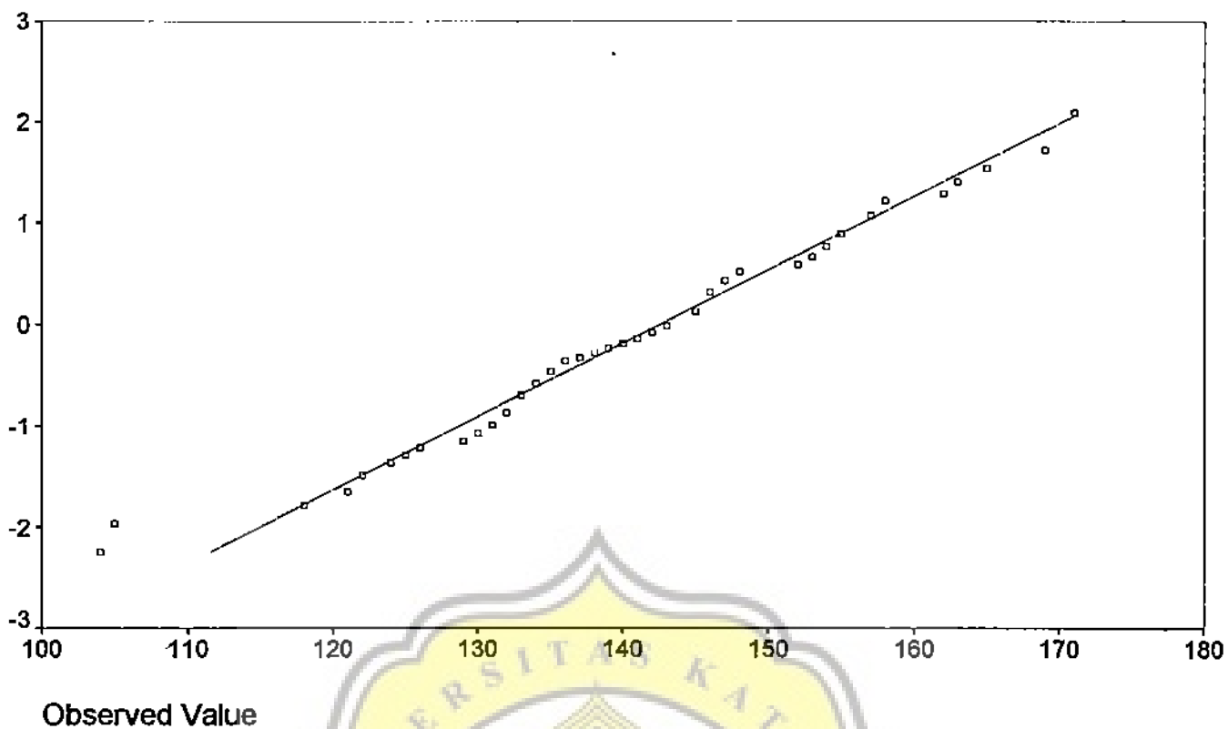
Normal Q-Q Plot of Intensitas Interaksi Teman Sebaya
